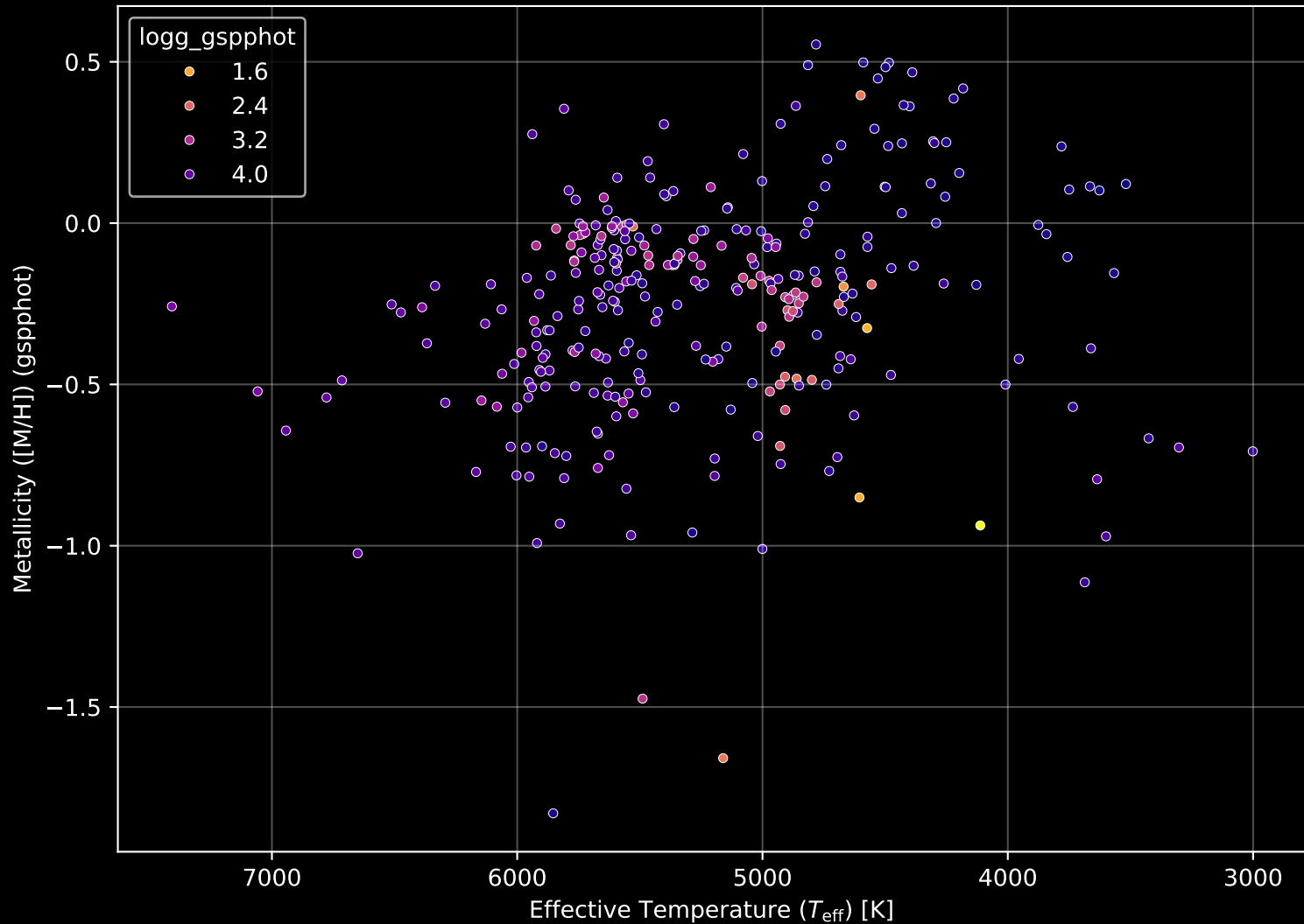
APOGEE DR17 Field: [293+62_btx] Stellar Population Parameters (n= 313)
